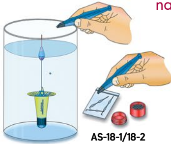
AS-18-1/18-2 Stonfo wyważarki do szaławików, 2 rozmiary.
